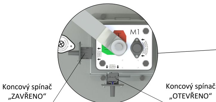
Provedení .80
