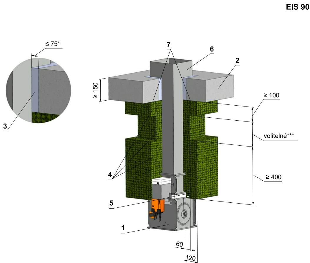
Obr. 46 Mimo tuhou stropní konstrukci - doizolace minerální vlnou - sádra nebo malta
