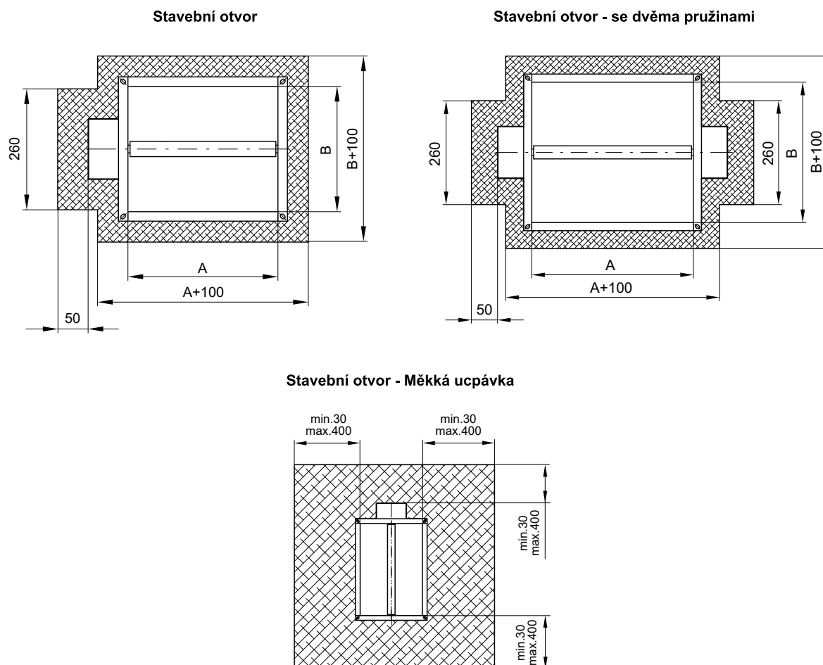
Obr. 27 Doporučené stavební otvory
