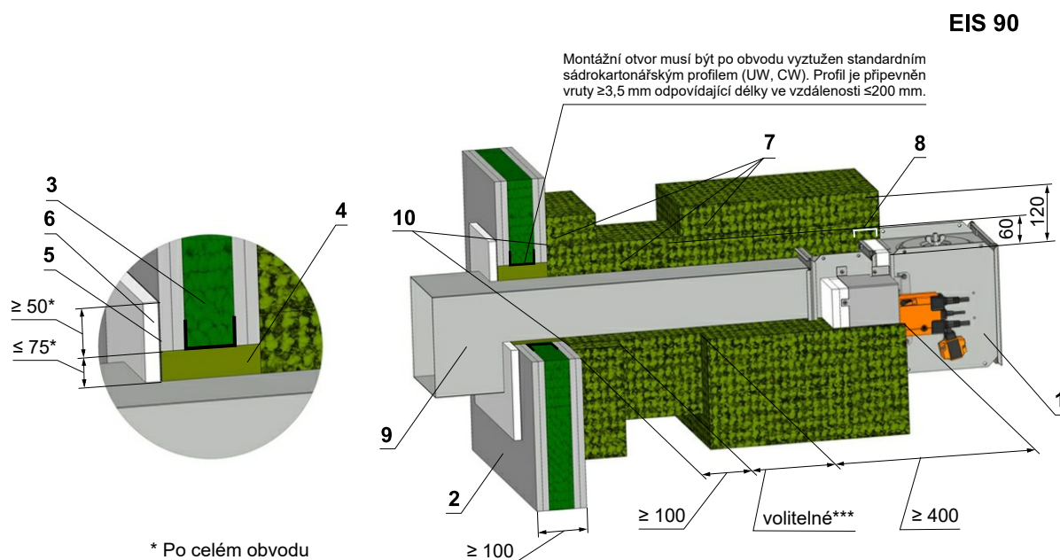
Obr. 42 Mimo sádkokartonovou konstrukci - doizolace minerální vlnou
