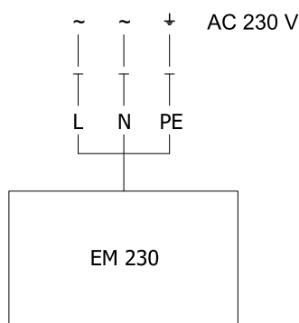
Obr. 7 Elektromagnet EM230
