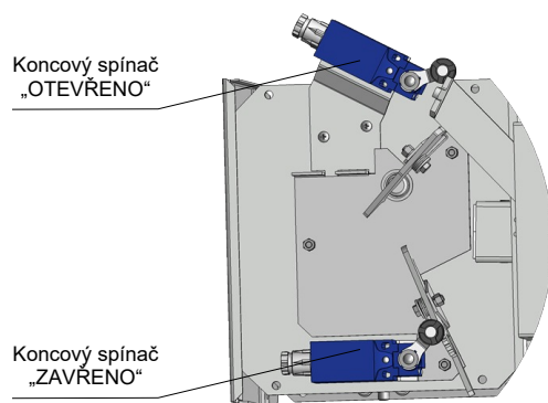
Obr. 10 Provedení .80 - provedení s mechanickým ovládáním a koncovým spínačem „OTEVŘENO“, „ZAVŘENO“
