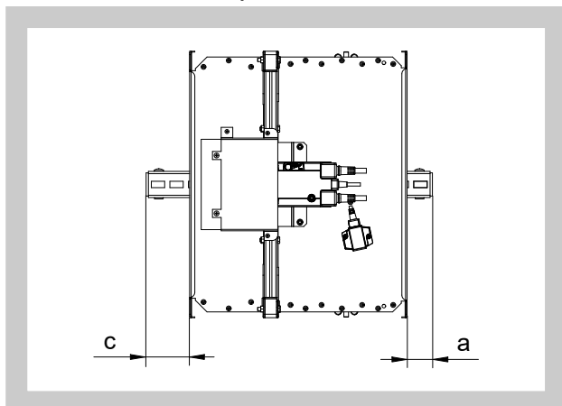
Obr. 23 Přesah klapky
