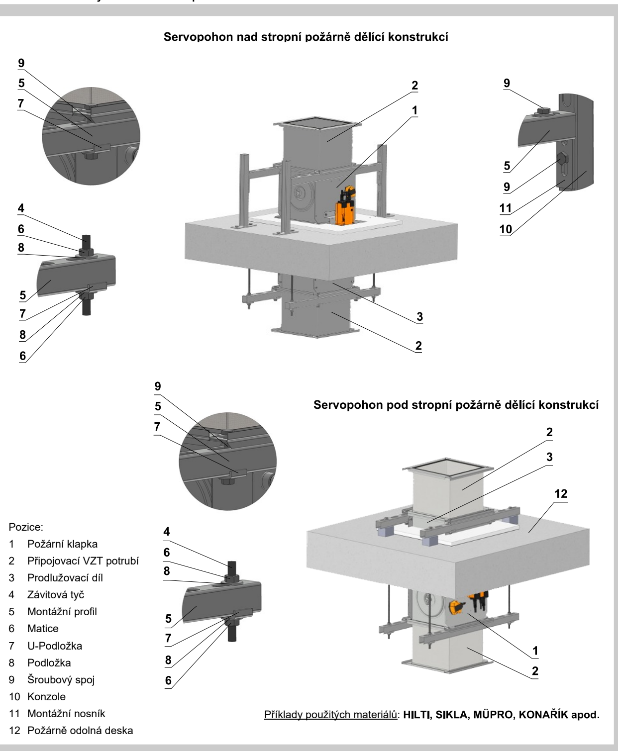
Obr. 51 Příklady zavěšení - svislé potrubí
