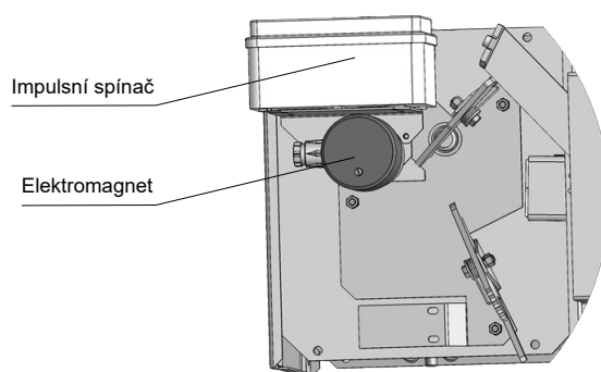
Obr. 6 Provedení .20, .21 - provedení s mechanickým ovládáním a elektromagnetem
