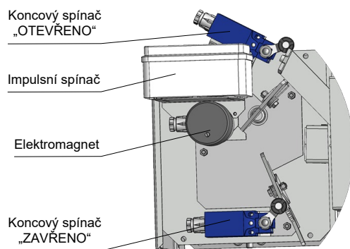
Obr. 11 Provedení .82, .83 - provedení s mechanickým ovládáním, koncovými spínači a elektromagnetem
