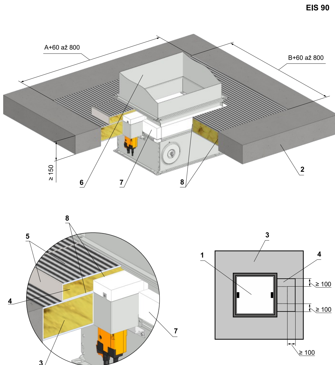
Obr. 45 Tuhá stropní konstrukce - měkká ucpávka
