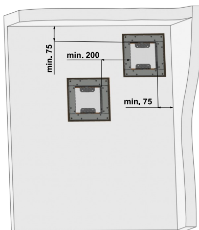
Obr. 25 Zabudování dvou a více klapky v jedné požárně dělící konstrukci
