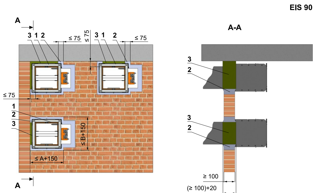
Obr. 30 Tuhá stěnová konstrukce - zabudování u stěny, stropu - sádra nebo malta a minerální vlna
