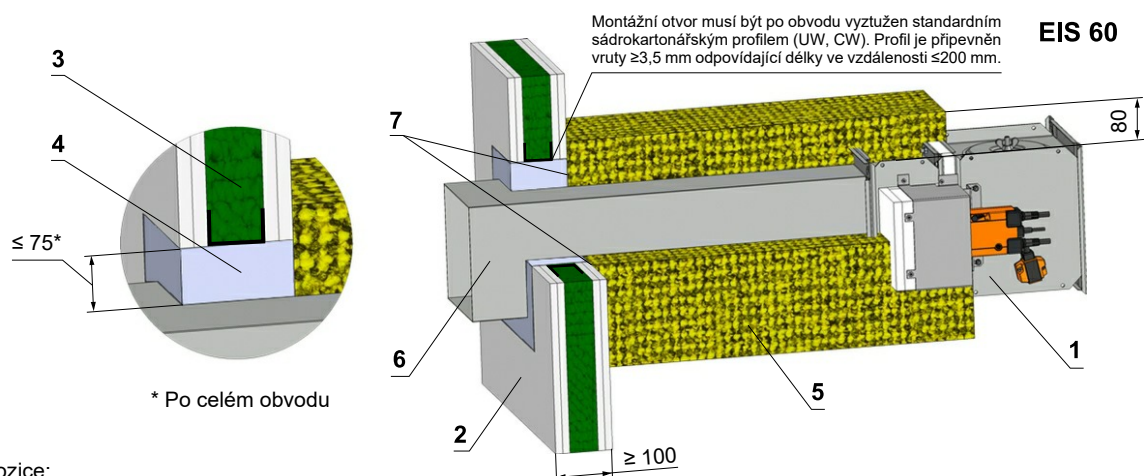
Obr. 40 Mimo sádkartonovou konstrukci - doizolace minerální vlnou - sádra nebo malta
