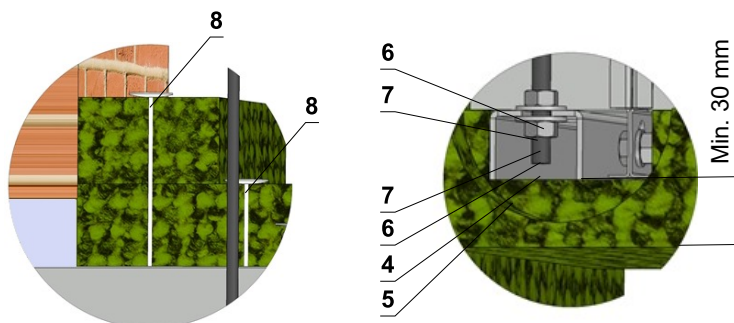
Umístění jednotlivých vrstev protipožární izolace na potrubí
