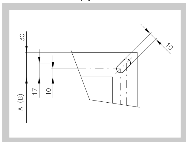
Obr. 24 Příruba klapky
