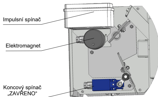
Obr. 9 Provedení .23, .24 - provedení s mechanickým ovládáním, koncovým spínačem a elektromagnetem
