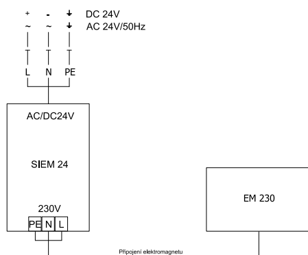
Obr. 8 Elektromagnet EM230 s impulsním spínačem SIEM24
