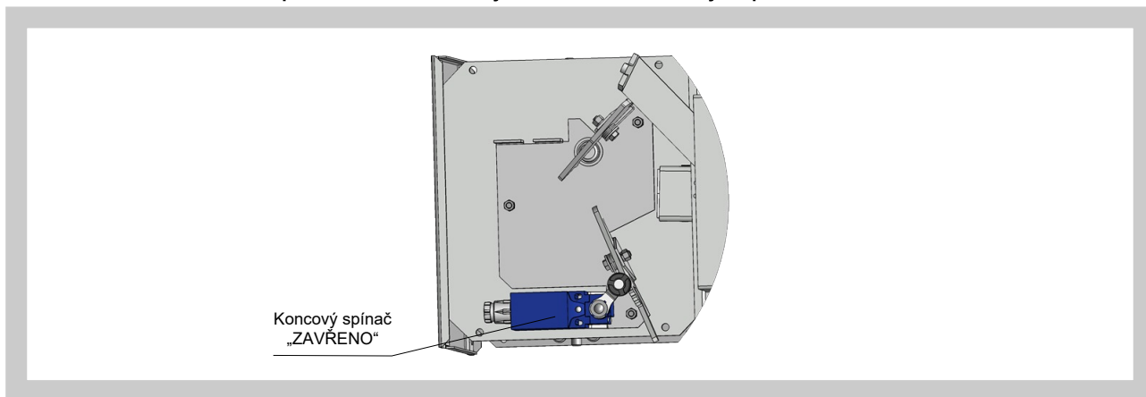
Obr. 5 Koncový spínač typu XCKN2118G-11
