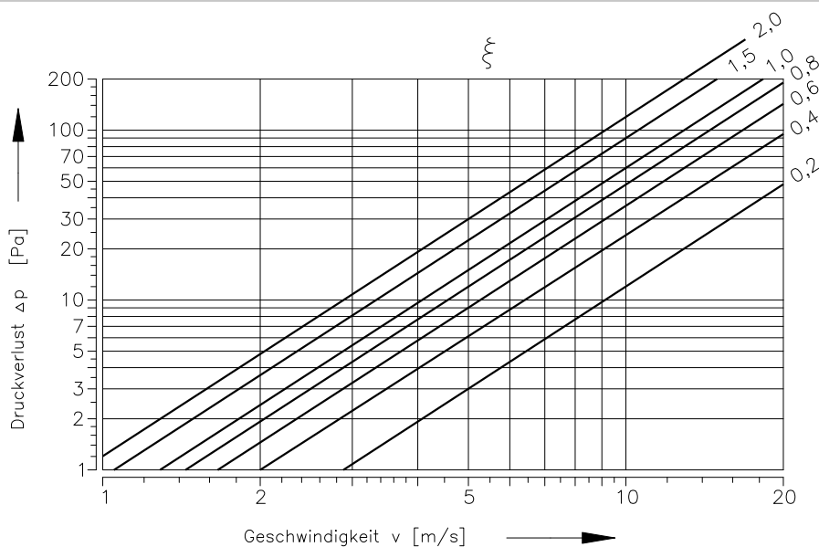
Diagramm 1. Druckverlust für die Luftdichte \rho = 1,2 \text{ kg/m}^3
