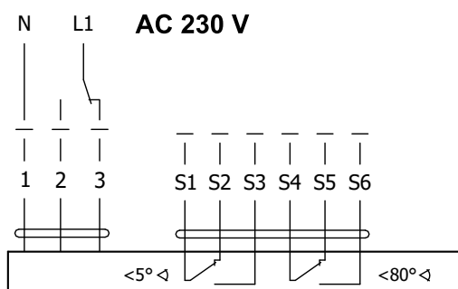
Abb. 7 Stellantrieb BELIMO BEN 230
