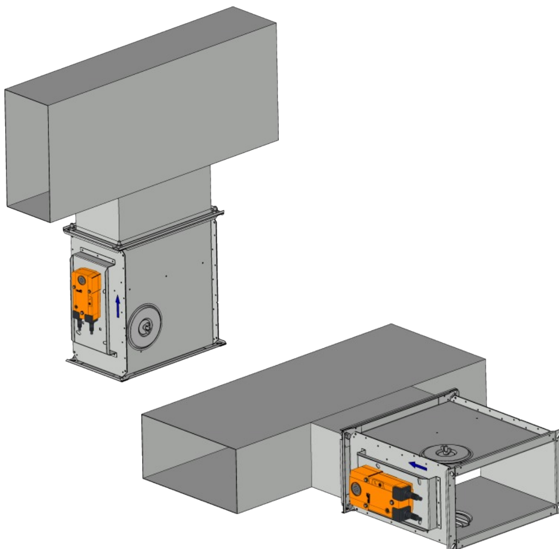
Abb. 4 Beispiele der Installation von Entrauchungsklappen
