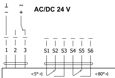
Abb. 8 Stellantrieb BELIMO BEE 24(-ST)
