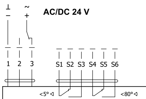
Abb. 6 Stellantrieb BELIMO BEN 24(-ST)
