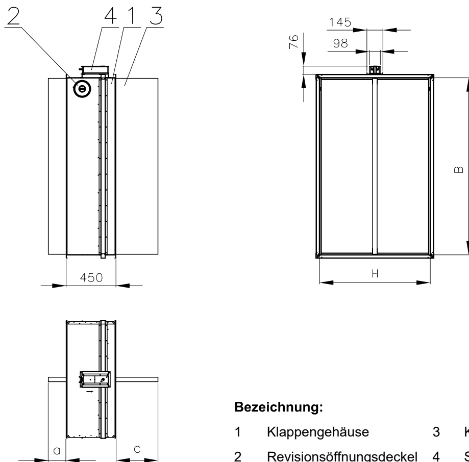
Abb. 2 Entrauchungsklappe - Single
