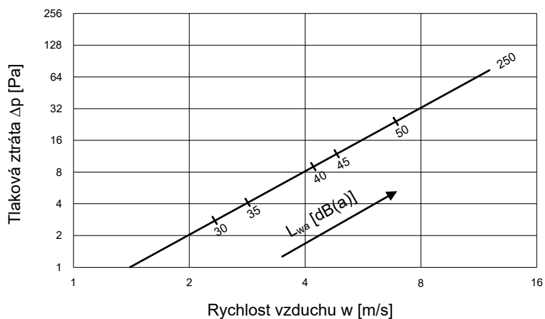
Diagram 1 Tlakové ztráty klapek pro hustotu vzduchu \rho = 1,2 \text{ kg.m}^{-3}
