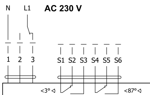
Abb. 10 Stellantrieb BELIMO BE 230-12
