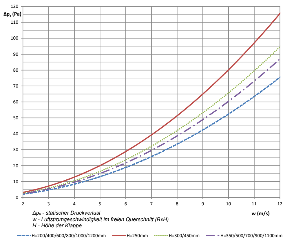
Diagram 1 Der Druckverlust für die Luftdichte 1,2 kg/m³
