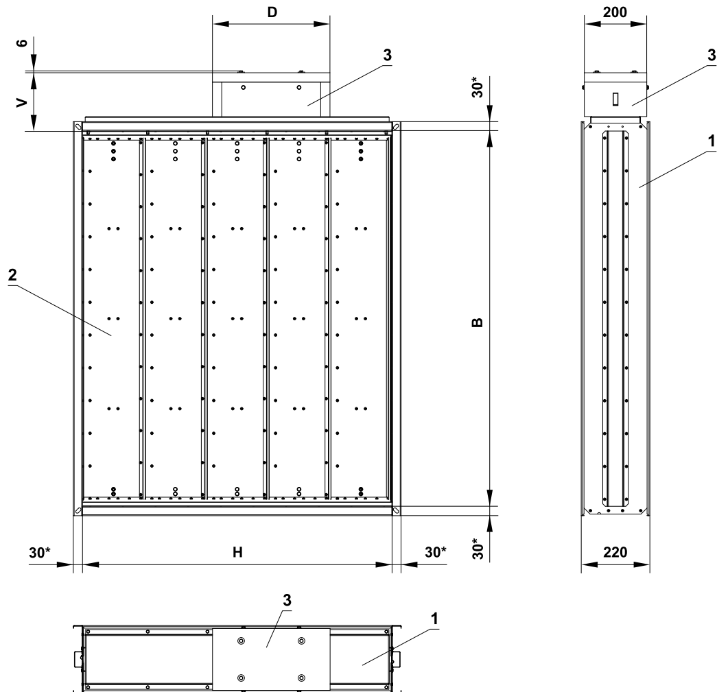
Abb. 11 Klappe SEDS-L
