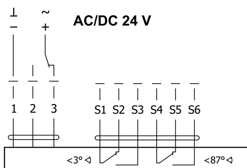
Abb. 9 Stellantrieb BELIMO BE 24-12(-ST)
