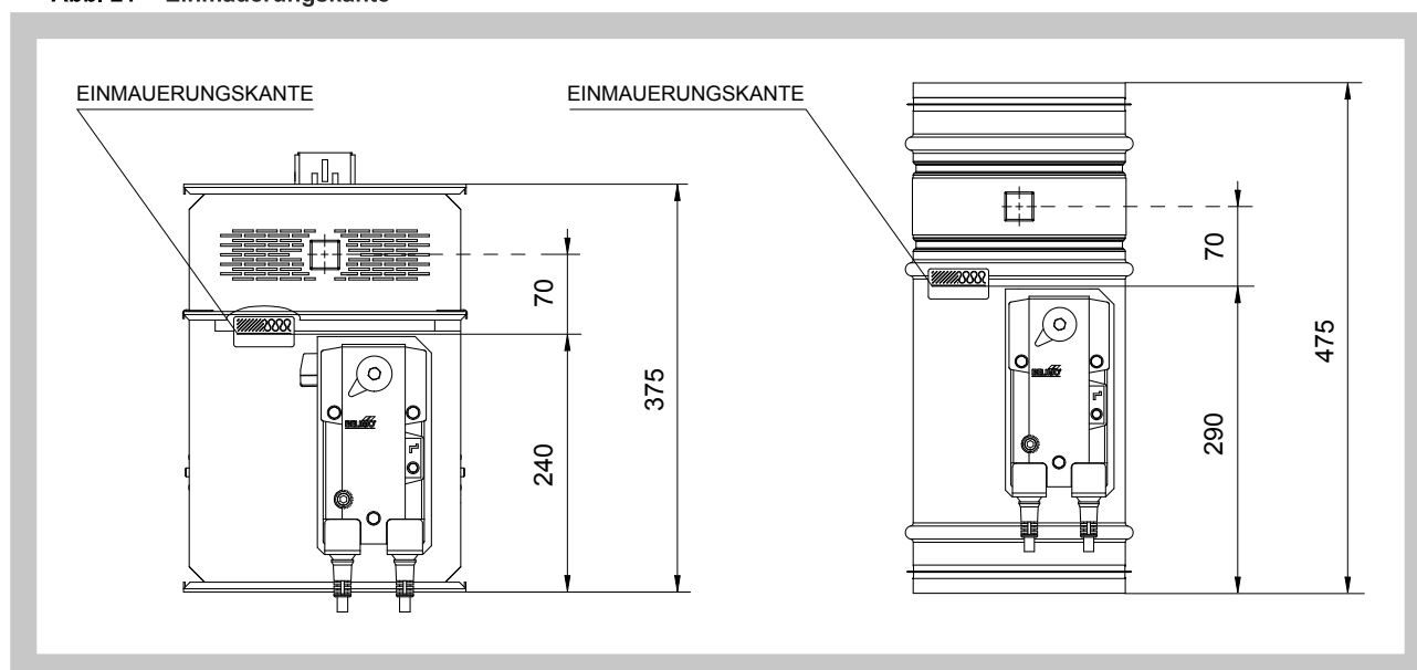
Abb. 21 Einmauerungskante
