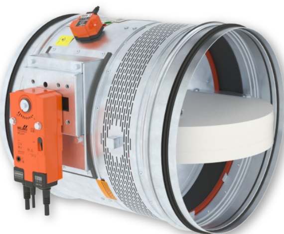
FDMR 180 se servopohonem
