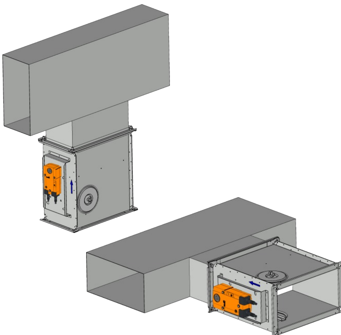
Obr. 5 Příklady instalace
