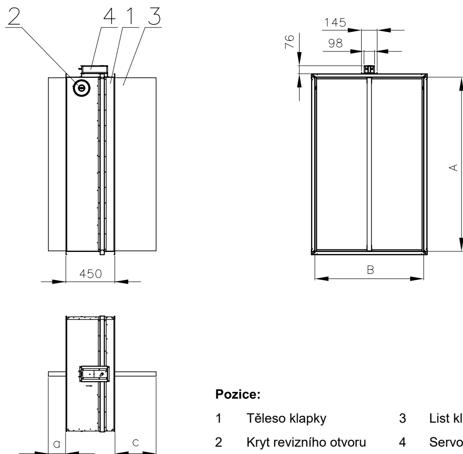
Obr. 3 Klapka odvodu kouře a tepla - single
