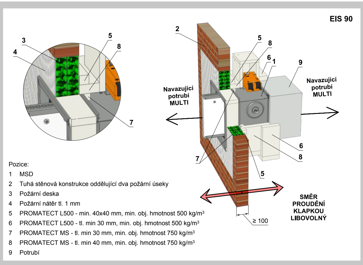
Obr. 39 Dělicí konstrukce mezi potrubím MULTI / MULTI - doizolace cementovápennými deskami - měkká ucpávka
