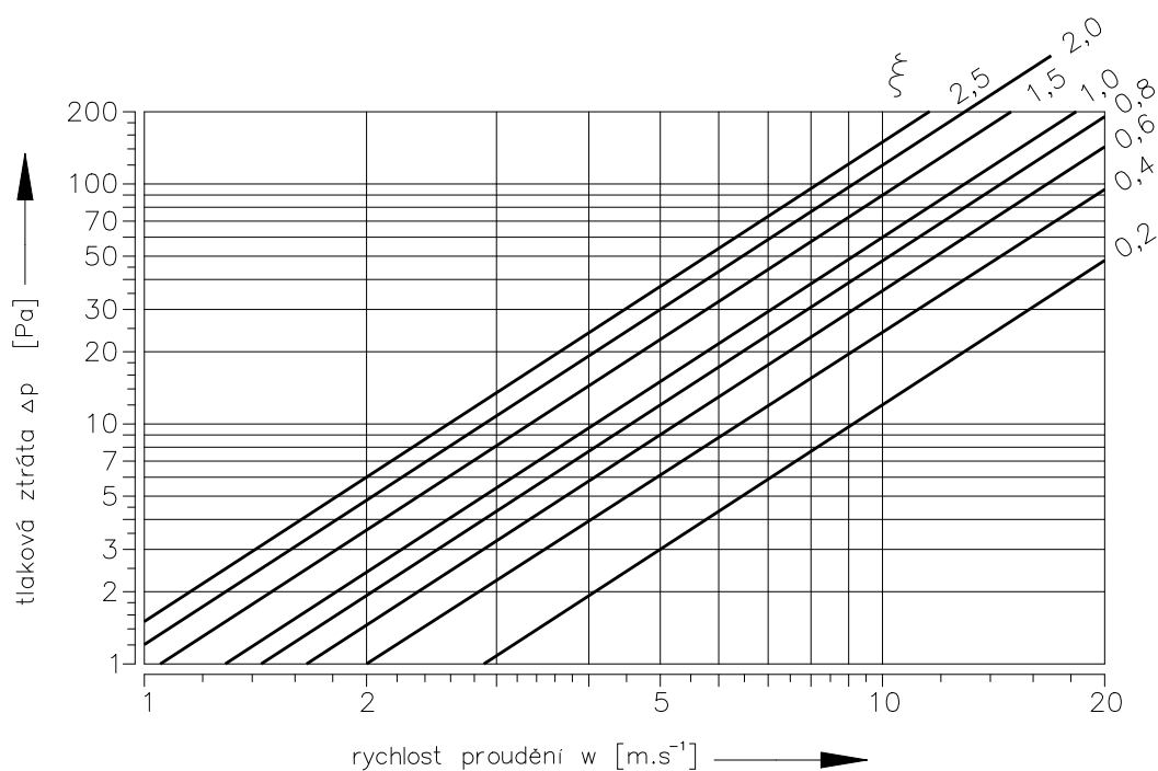
Diagram 6.2.1. Tlaková ztráta pro hustotu vzduchu
