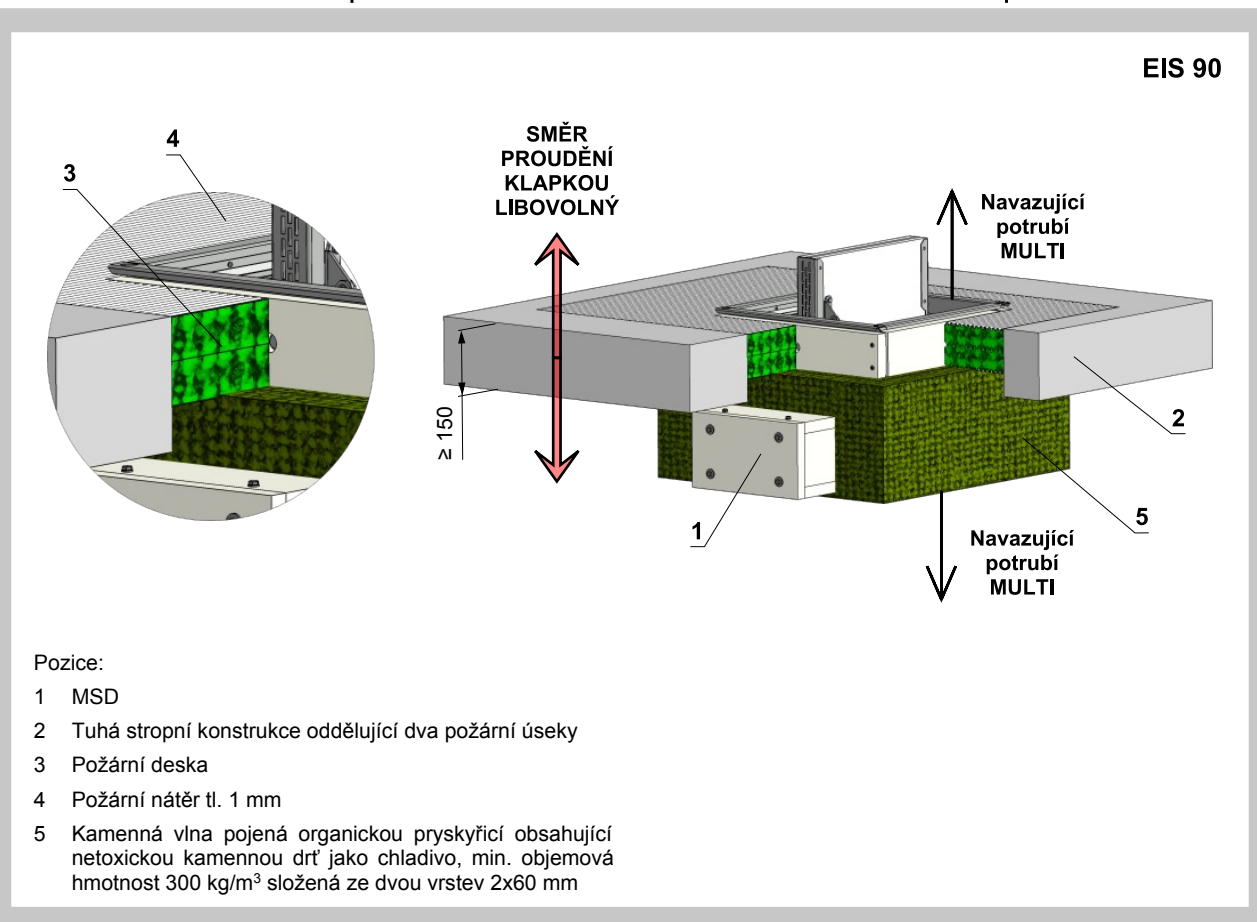
Obr. 52 Dělicí konstrukce mezi potrubím MULTI / MULTI - doizolace kamennou vlnou - měkká ucpávka
