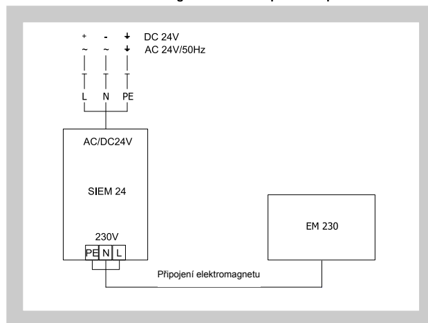
Obr. 18 Elektromagnet EM230 s impulsním spínačem SIEM24
