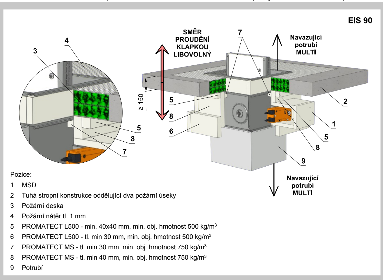
Obr. 53 Dělicí konstrukce mezi potrubím MULTI / MULTI - doizolace cementovápennými deskami - měkká ucpávka
