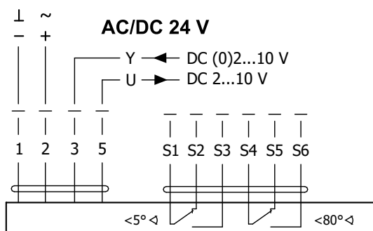
Obr. 5 Servopohon BELIMO BEN 24-SR - pouze u čtyřhranných klapek MSD
