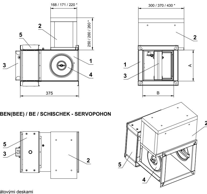
Obr. 22 Čtyřhranná MSD - provedení se servopohonem a boxem
