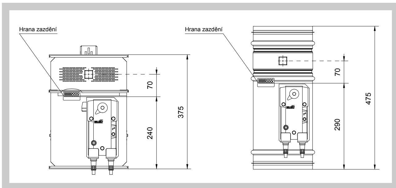
Obr. 29 Hrana zazdění
