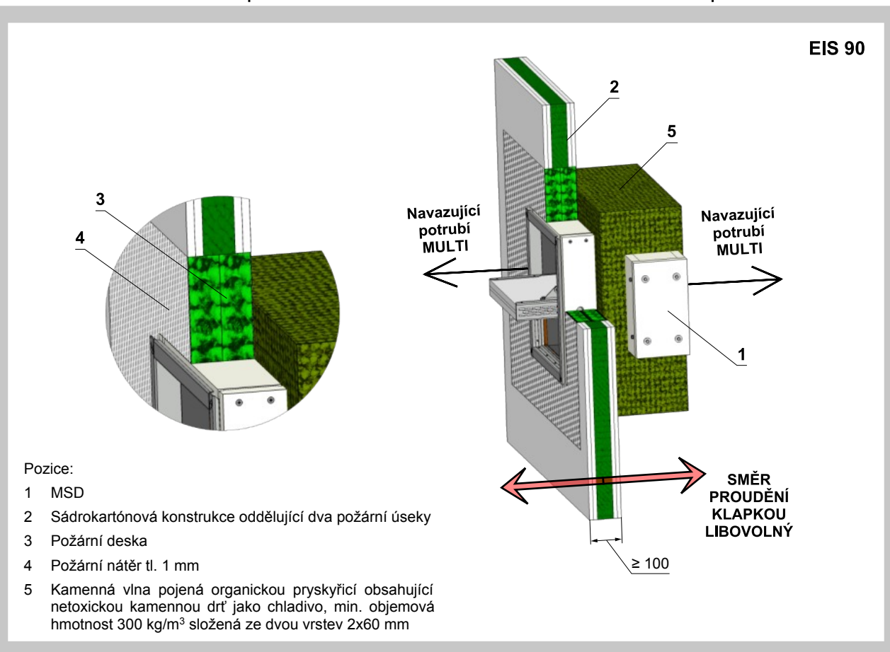
Obr. 45 Dělicí konstrukce mezi potrubím MULTI / MULTI - doizolace kamennou vlnou - měkká ucpávka
