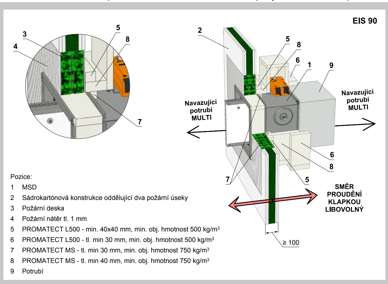
Obr. 46 Dělicí konstrukce mezi potrubím MULTI / MULTI - doizolace cementovápennými deskami - měkká ucpávka
