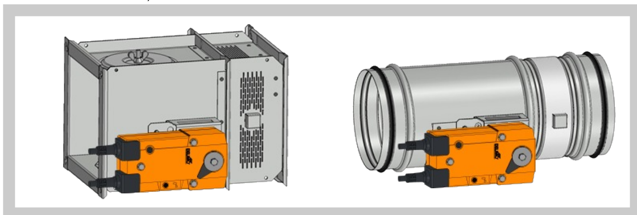
Obr. 3 Provedení .44, .54 a .65
