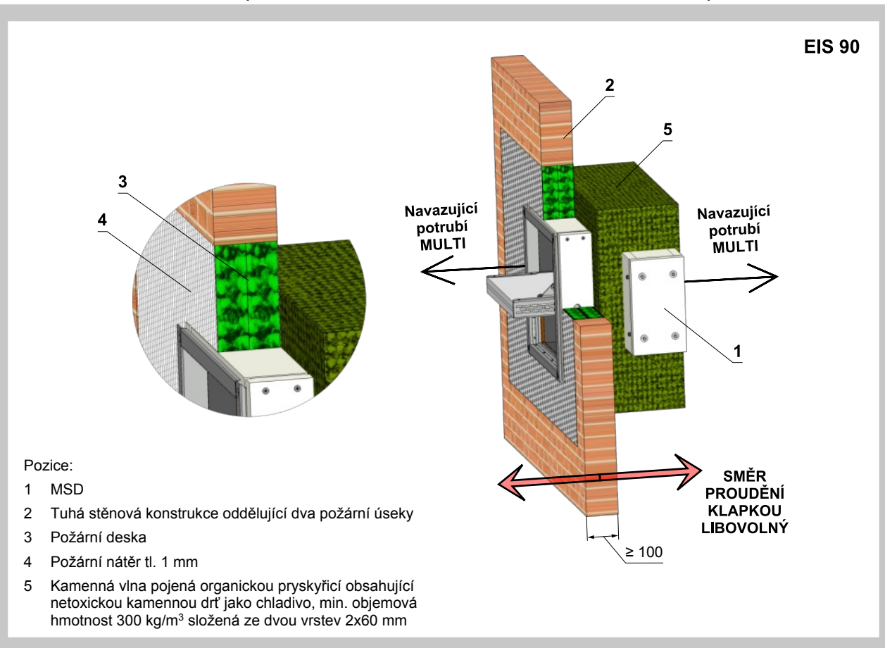
Obr. 38 Dělicí konstrukce mezi potrubím MULTI / MULTI - doizolace kamennou vlnou - měkká ucpávka
