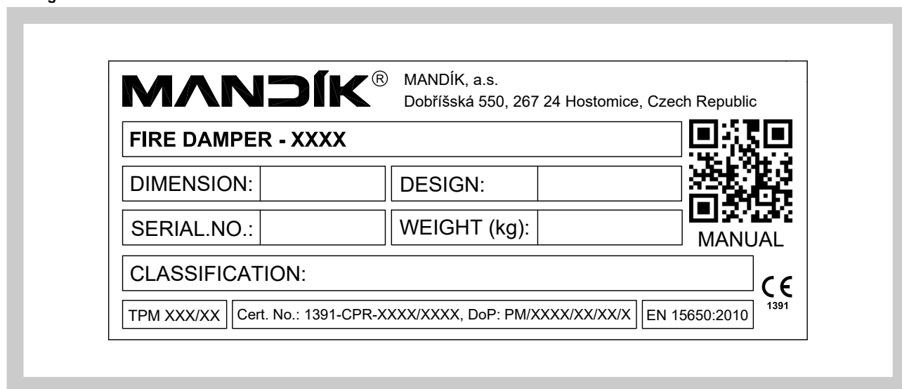
Fig. 54 Data label
