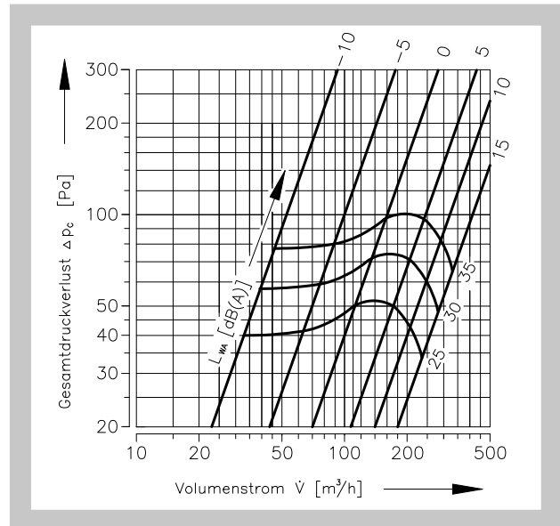
Diagramm 4 Zuluftventil TVPM 160
