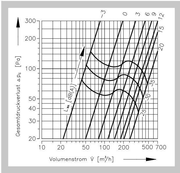
Diagramm 5 Zuluftventil TVPM 200
