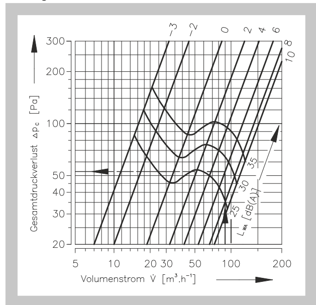
Diagramm 2 Zuluftventil TVPM 100
