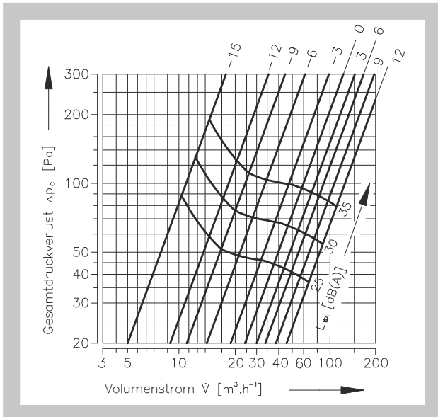
Diagramm 8 Abluftventil TVOM 125
