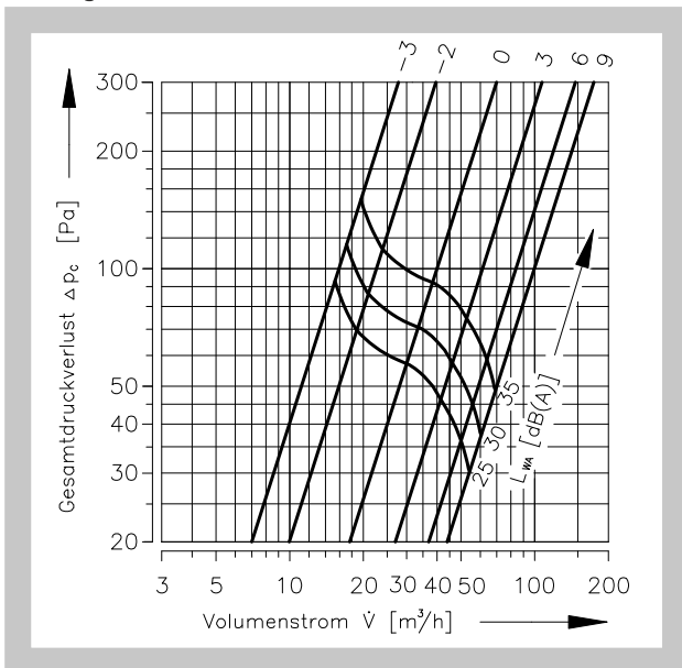
Diagramm 1 Zuluftventil TVPM 80
