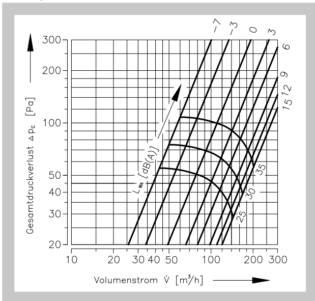
Diagramm 3 Zuluftventil TVPM 125
