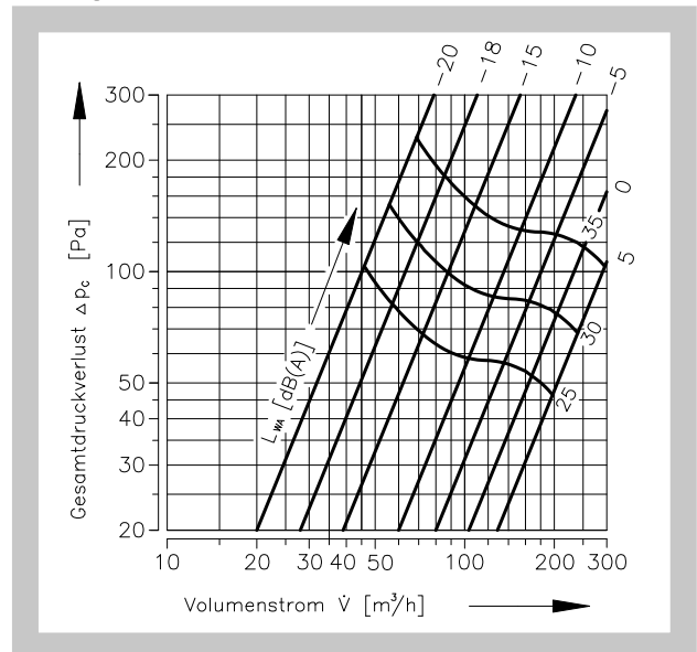
Diagramm 9 Abluftventil TVOM 160
