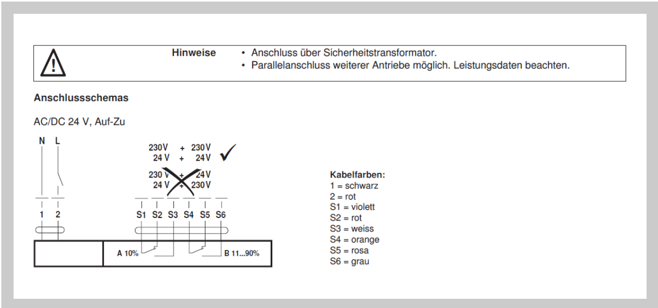
Abb. 21 Anschlussschema der Servoantriebe Belimo NFA-S2, SFA-S2
