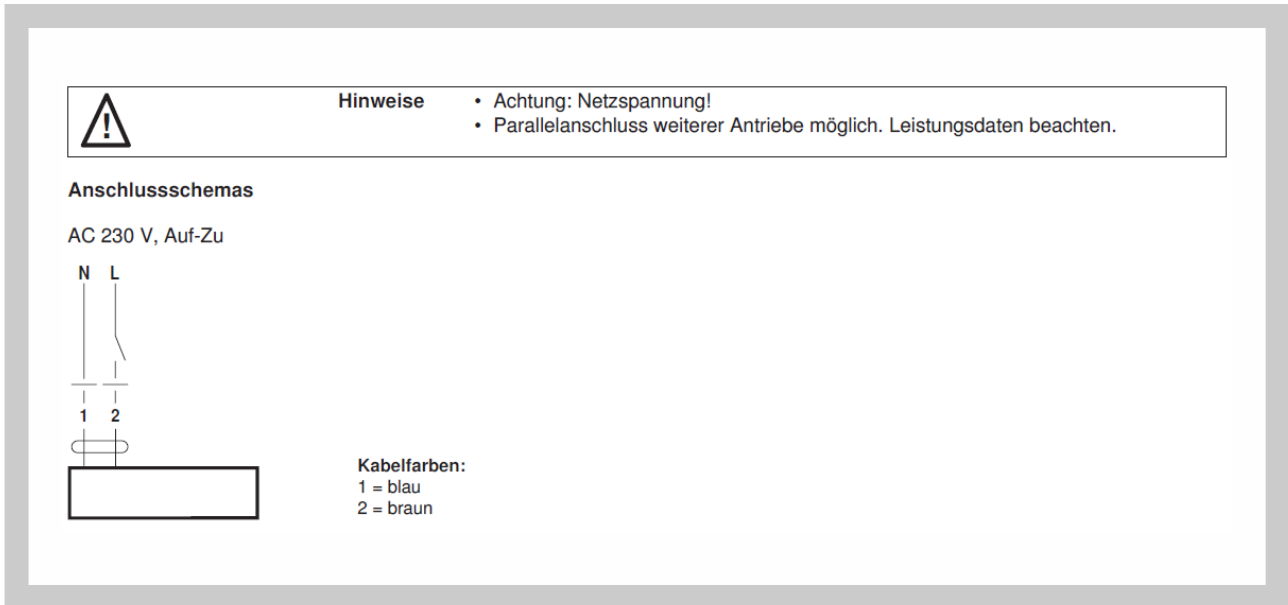
Abb. 17 Anschlussschema der Servoantriebe Belimo TF24-S, LF 24-S
