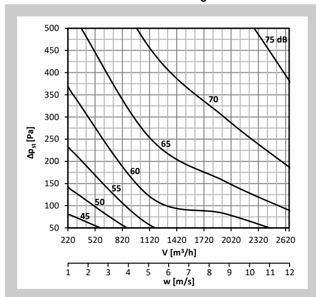
Diagramm Nr. 12 Schalleistungspegel L_{WA} [dB(A)] innerhalb der Anschlussleitung - DN355
