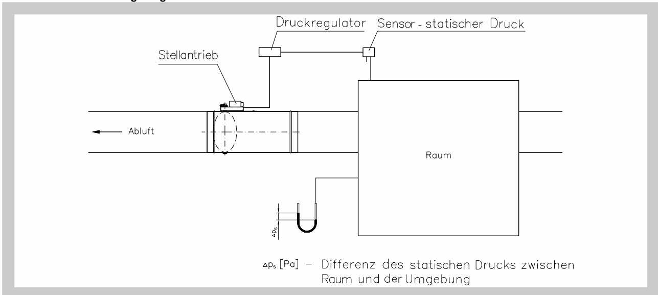
Abb. 5 Raumdruckregelung
