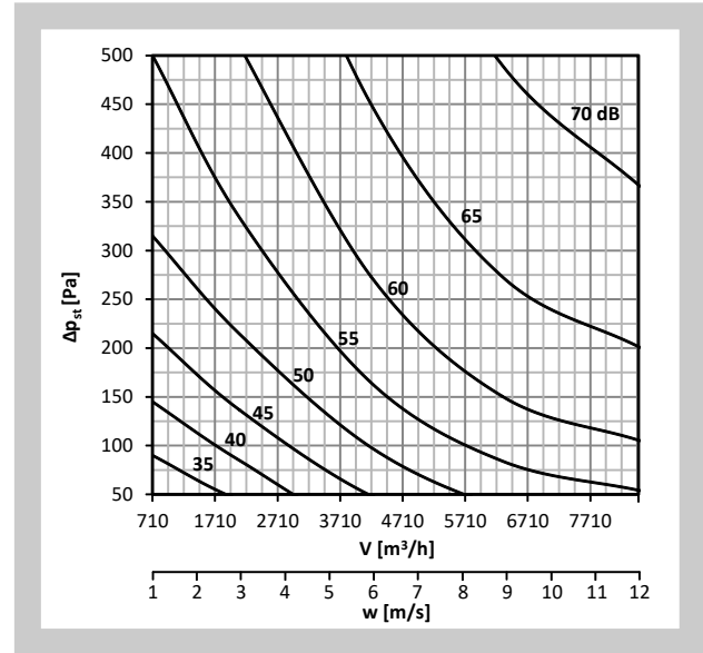
Diagramm Nr. 29 Schalleistungspegel L_{WA} [dB(A)] außerhalb der Anschlussleitung - DN500, nicht isoliert
