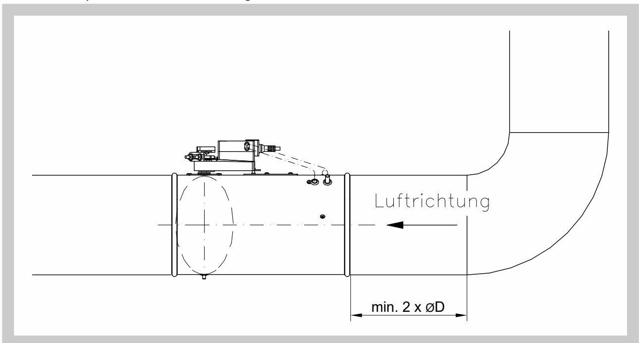
Abb. 32 Empfohlener Abstand vom Rohrbogen
