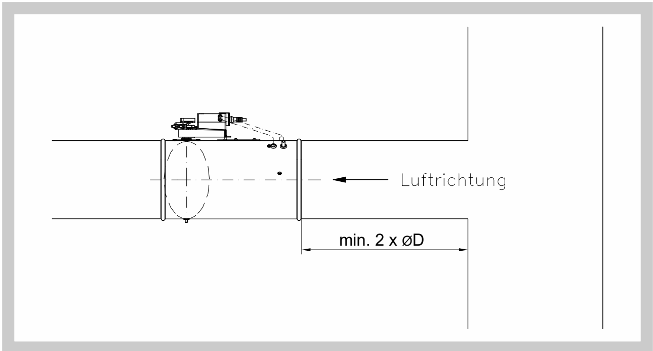
Abb. 31 Empfohlener Abstand vom Verteiler
