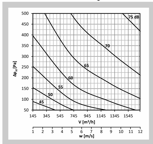
Diagramm Nr. 10 Schalleistungspegel L_{WA} [dB(A)] innerhalb der Anschlussleitung - DN280
