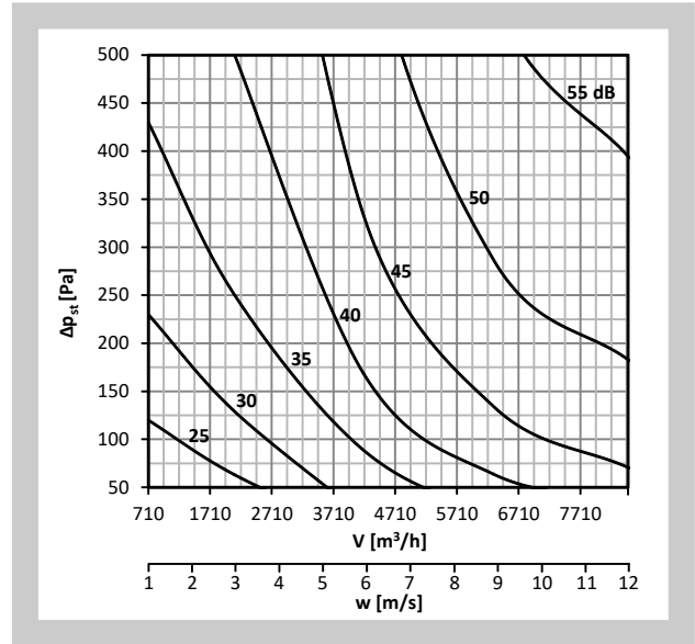
Diagramm Nr. 44 Schalleistungspegel L_{WA} [dB(A)] außerhalb der Anschlussleitung - DN500, isoliert
