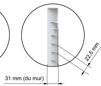
Détail A - coupe transversale
