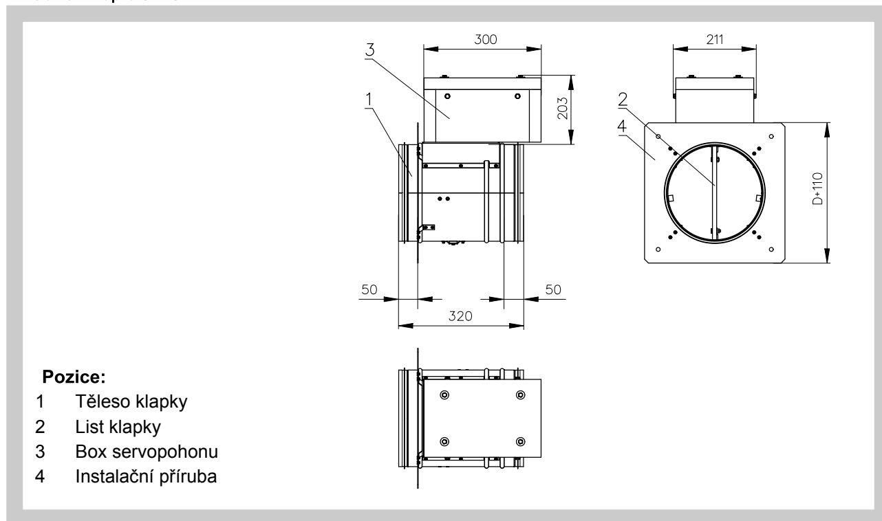
Obr. 8 Klapka SEDS-R
