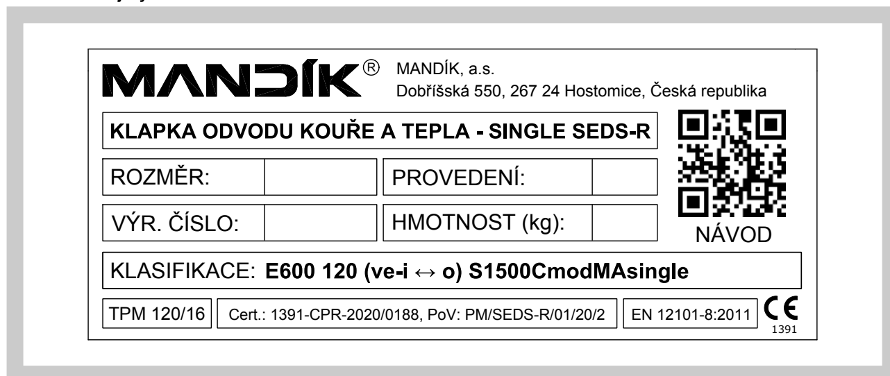
Obr. 11 Údajový štítek
