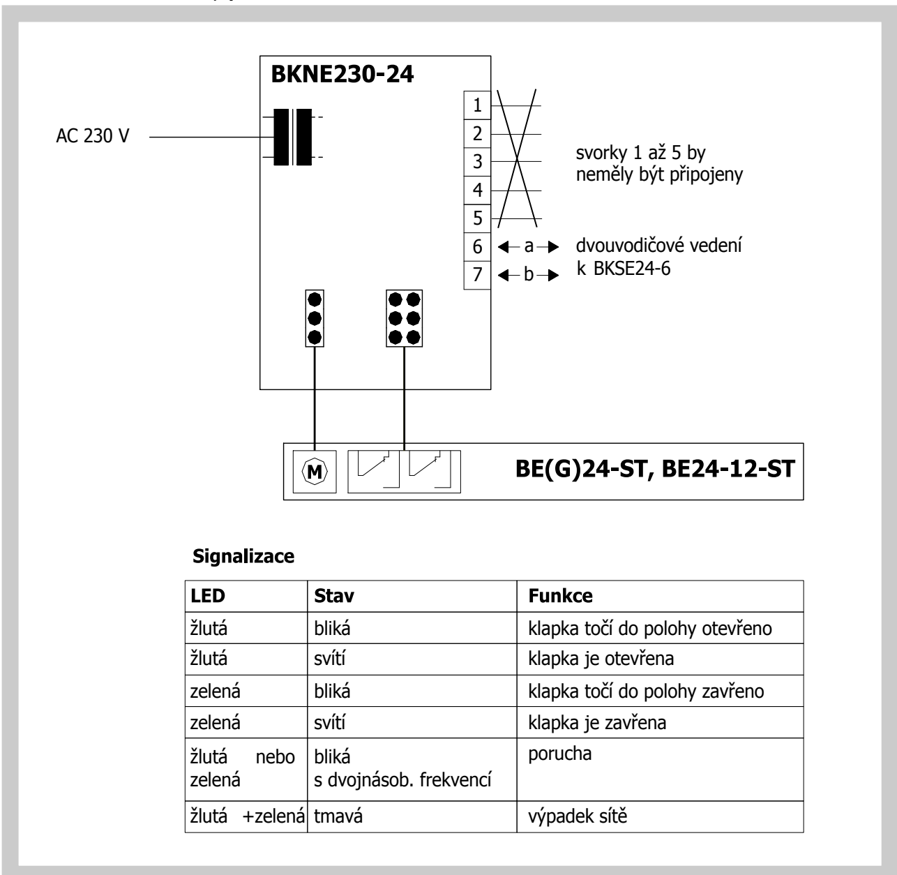
Obr. 6 Komunikační a napájecí zařízení BKNE 230-24
