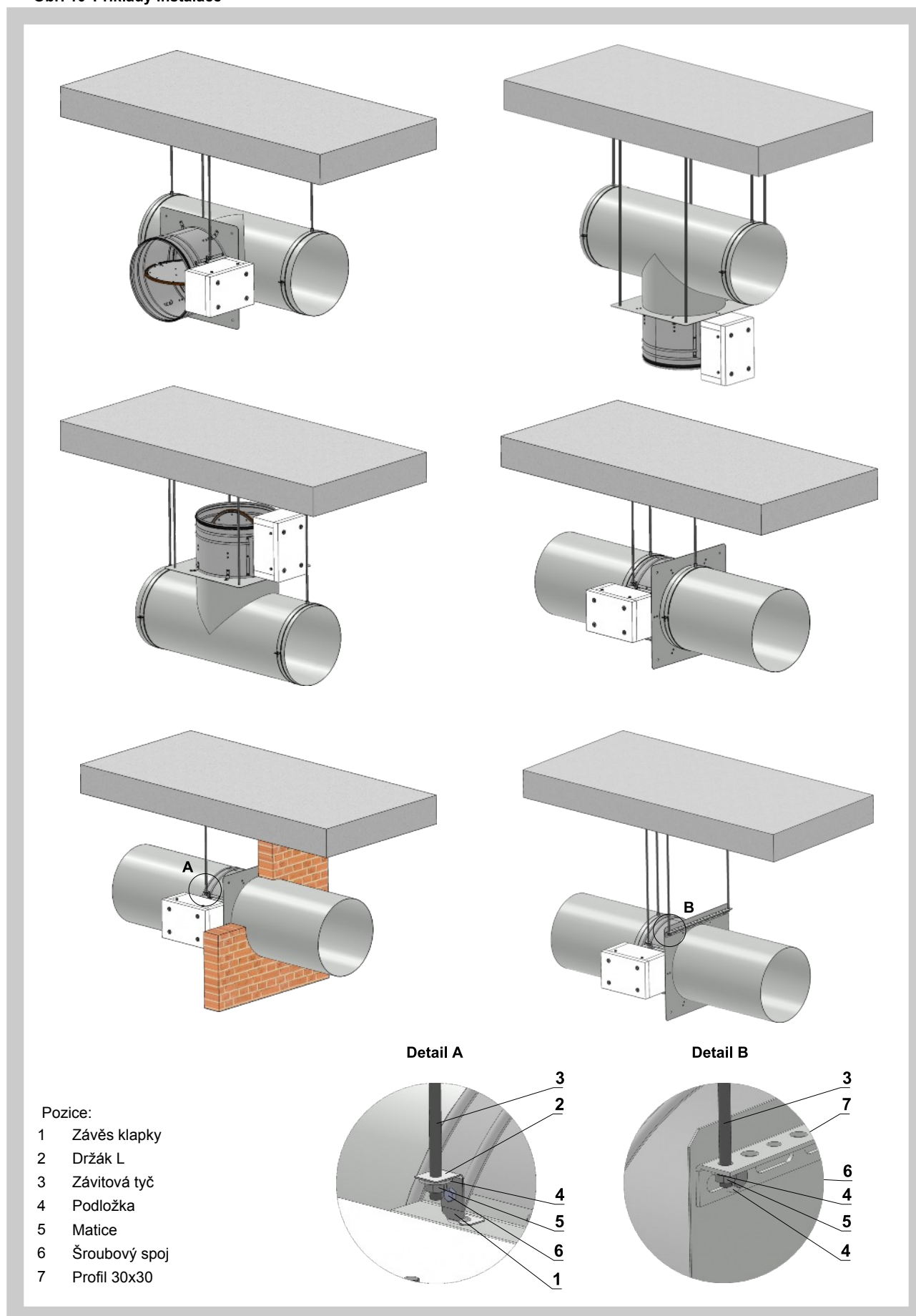
Obr. 10 Příklady instalace
